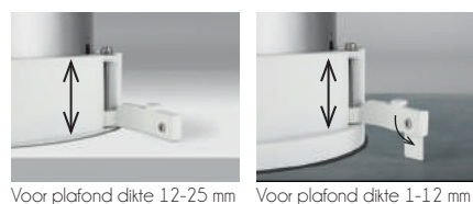
Voor plafond dikte 12-25 mm
