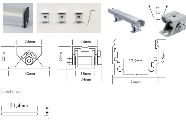
Schuifbasis
