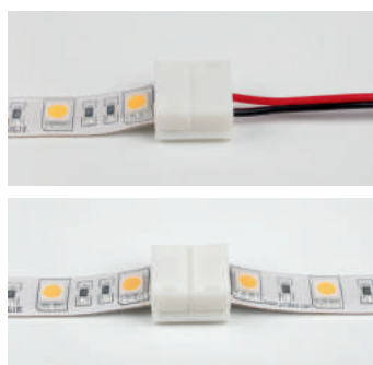
Easy Connect Systeem voor IP53 Mono 10mm*
