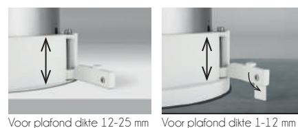
Voor plafond dikte 12-25 mm Voor plafond dikte 1-12 mm
