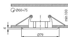
Zaagmaat Ø60-7
