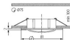
Zaagmaat Ø75
