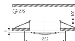
Zaagmaat Ø75
