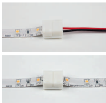
Easy Connect Systeem voor IP53 Mono 8mm*
