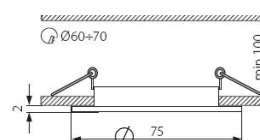
Zaagmaat Ø60-70
